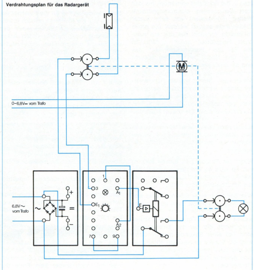
Verdrahtungsplan für das Radargerät
