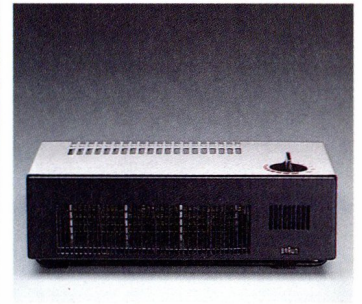
Braun Heizlüfter H 10 Leistungsstarker Heizlüfter mit stufenlos einstellbarem Thermostat für konstante Raumtemperatur. 3 Heizstufen und zusätzliche Kaltstufe, alle Funktionen mit einem Schalter zu bedienen.
