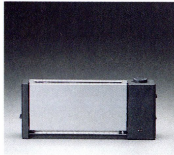
Braun Toaster HT 6 Zweischeiben-Toastautomat für viele Brotsorten. Die pneumatische Auswurfmechanik drückt den fertigen Toast nach oben und vermeidet ein Herauspringen der Scheibe.
