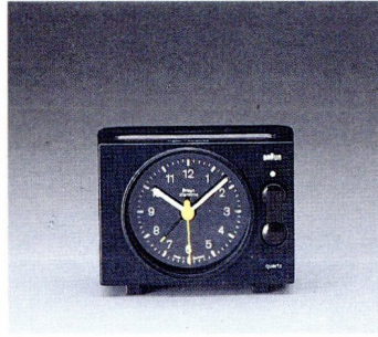
Braun sensormat® quartz AB 20 sl Batterie-Weckuhr mit extrem leisem Lauf durch Braun silentime quartz Uhrwerk. Hoher Bedienungskomfort durch Sensortaste für Nachweckfunktion und Zifferblattbeleuchtung. Anschwellender Weckton.
