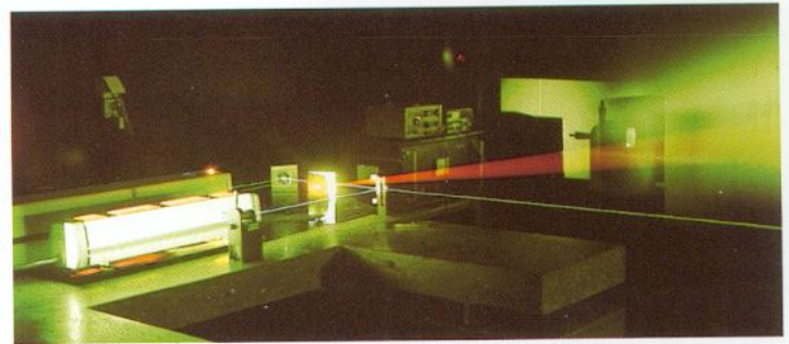
Hologramme werden mit Laserlicht fotografiert. Hier ein Laboraufbau.
