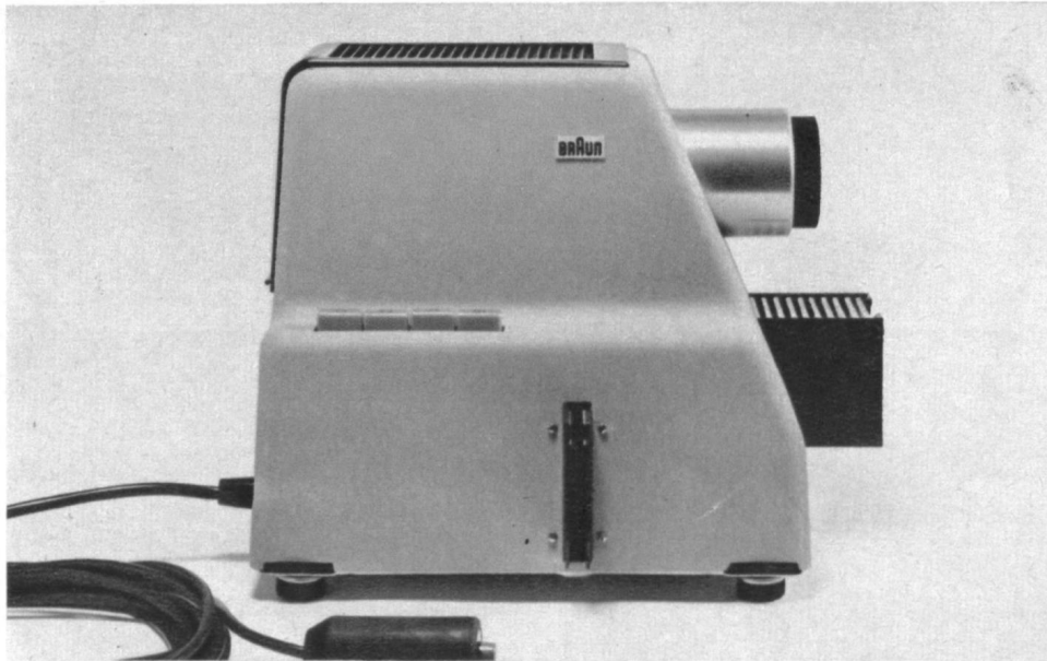
Automatischer Kleinbildprojektor PA 2 mit ferngesteuertem Bildwechsel; Farbkorrigiertes Isco-Objektiv der Lichtstärke 1:2,8; Kamin-Konvektionskühlung. Mit Magazin, Fernbedienungskabel und Lampe DM 230.—
