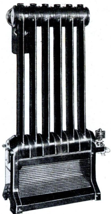
Element-Gas-Ofen mit offenem Flammenraum für alle Zwecke
