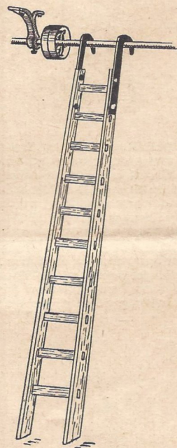
Nr. 160 Transmissionsleiter , Holme aus sauberer Blockware, besonders kräftig, senkrecht stehende Hartholzsprossen, beiderseitig verleimt und doppelt verkeilt. Einhängenhaken werden nur nach besonderer Bestellung und Angabe von gewünschten Maßen angefertigt. Sprossenabstand 28 cm.
