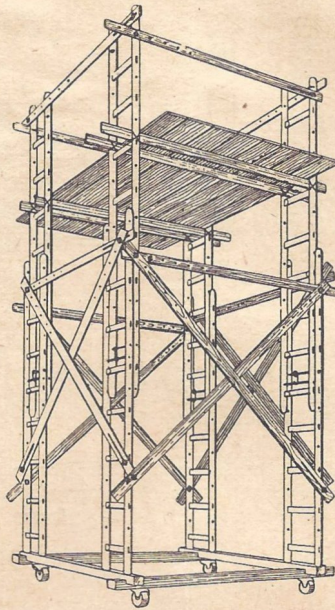
Fahrbares Deckengerüst
