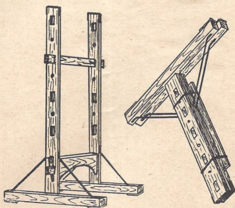
Nr. 122 Gerüstbock , besonders für schwere Arbeiten geeignet, in verschiedenen Abmessungen, leicht aufzubauen und auf kleinstem Raum zu lagern.
