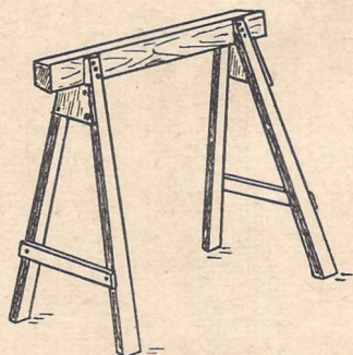
Nr. 121 Tapezierbock , feststehend, Füße eingezapft und mit durchgehenden Schloßschrauben verschraubt sowie doppelt verstrebt.
