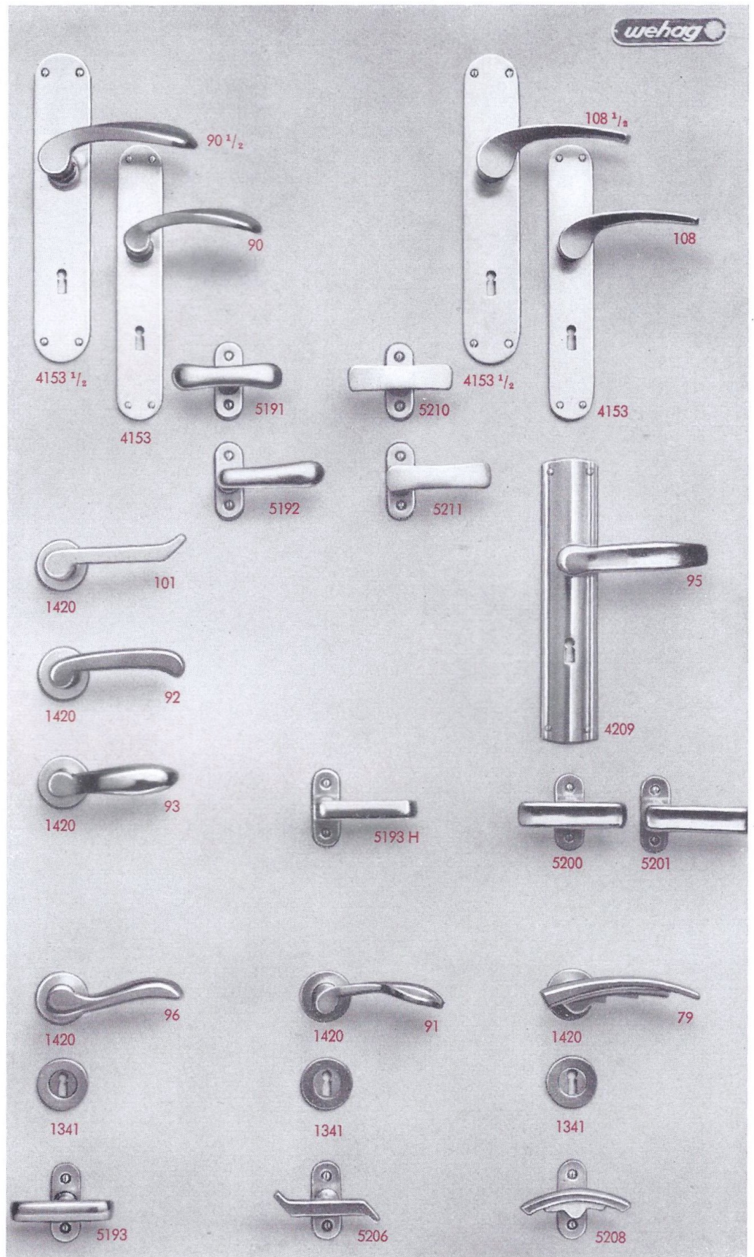
Wehag-Leichtmetall eloxierte Türdrücker mit Langschildern Türdrücker mit Rosetten und Schlüsselschildern Fensteroliven
