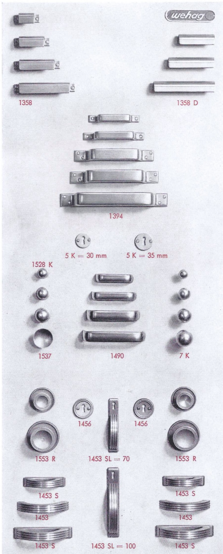
Wehag-Leichtmetall eloxierte Möbelgriffe, Möbelknöpfe und Schlüsselschilder
