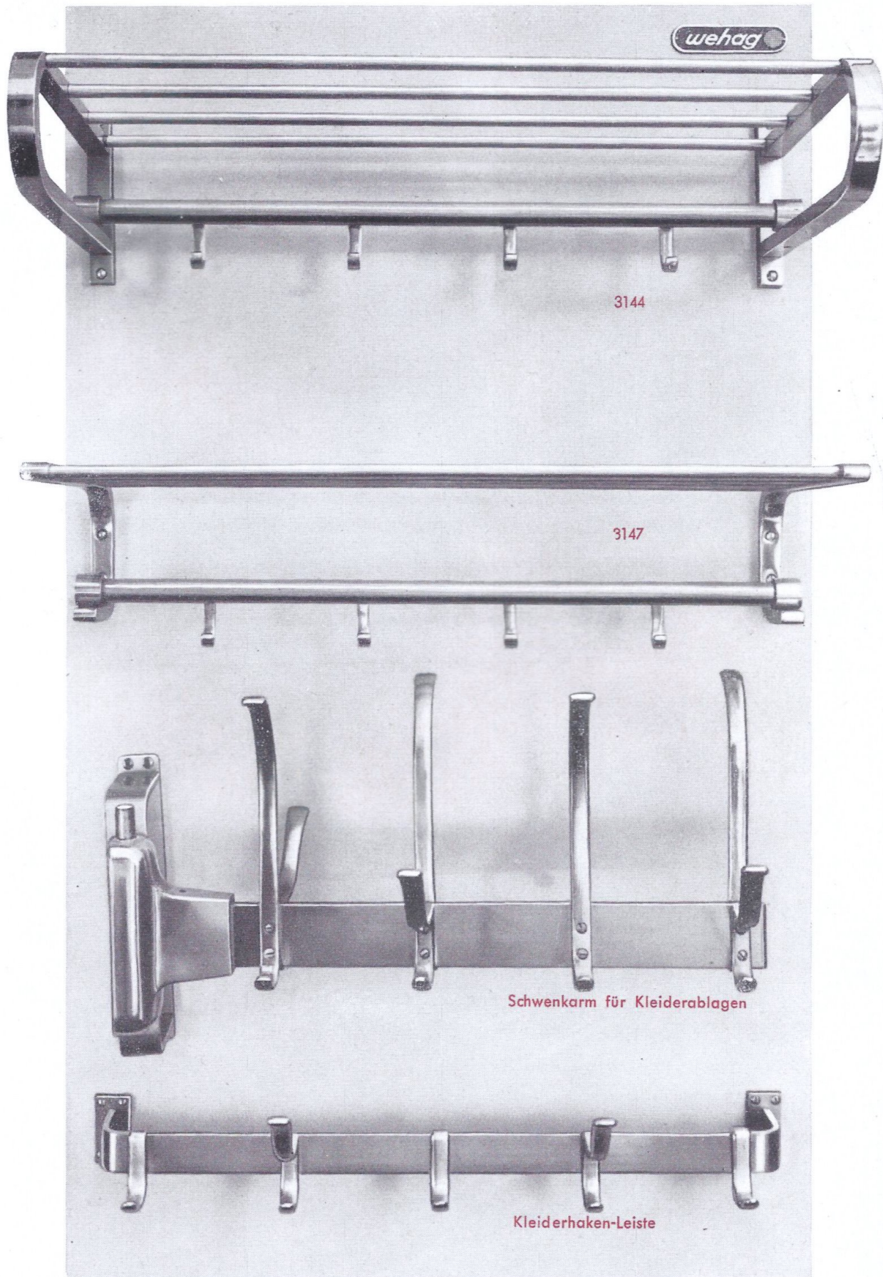
Wehag-Leichtmetall eloxierte Kleiderablagen, Schwenkarme für Kleiderablagen und Kleiderhaken-Leiste, in verschiedenen Längen lieferbar
