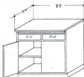
Küchentisch KTK
