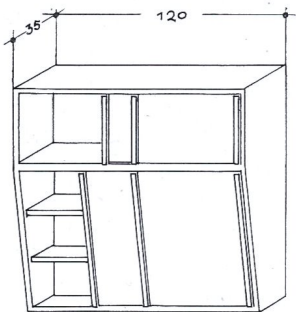
Wandschrank HBS
