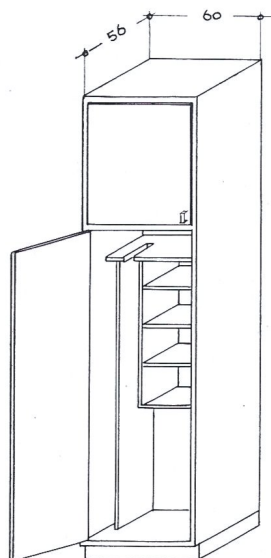
Besenschrank BSN
