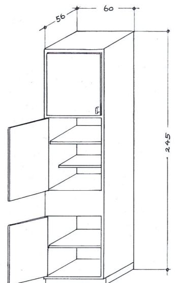
Küchenschrank KSK
