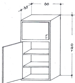
Wandschrank HSG
