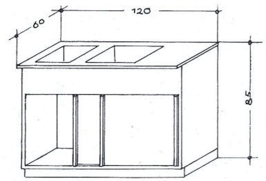
Spültischunterbau SU
