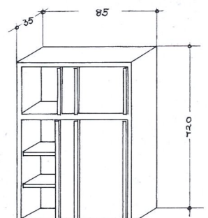
Wandschrank WGS
