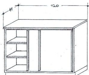
Küchentisch KTS
