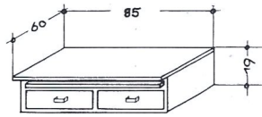
Küchentisch KZT
