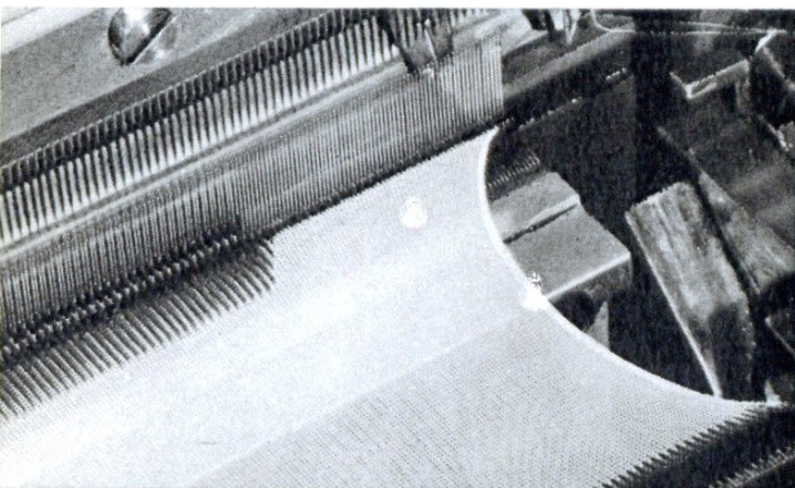
Flachwirk-Maschine (Ausschnitt)
