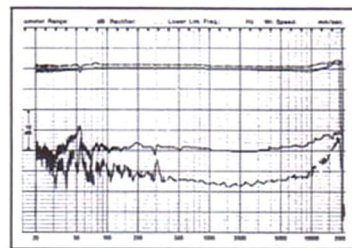
Frequenzgang des linken und rechten Kanals sowie die Stereo-Übersprechdämpfung
