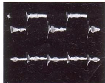
Rechteckwiedergabe des Tonabnehmers; oben Summe aus rechtem und linkem Kanal, unten Differenz
