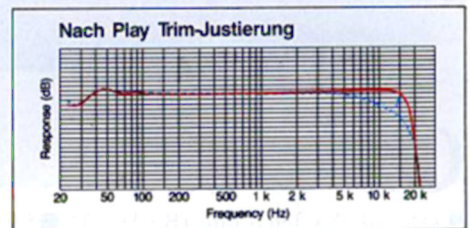
Effekt der Play Trim-Justierung
