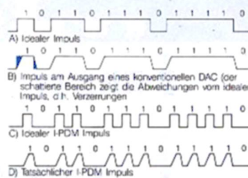
Das I-PDM-System
