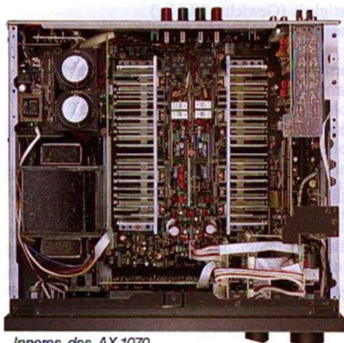
Inneres des AX-1070
