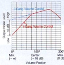
Ausgangsrauschen (4- und 2-stufiger Lautstärkereger)
