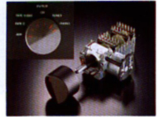
Motorbetriebener Eingangswahlschalter
