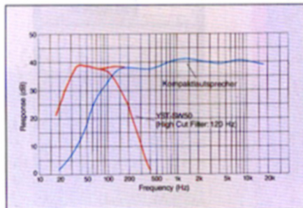
Frequenzgang (YST-SW50 + Kompaktlautsprecher)
