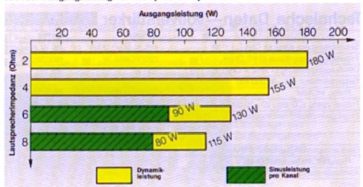
RX-750: Ausgangsleistung vs. Lautsprecherimpedanz
