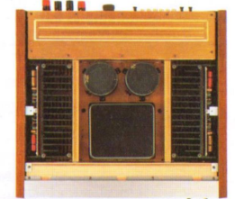
Inneres des AX-2000
