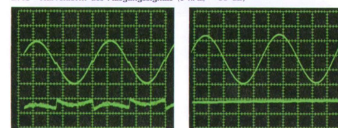
Herkömmlicher D/A-Konverter (Ladder Typ)
