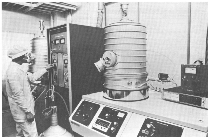
Beryllium Verdampfungs Anlage
