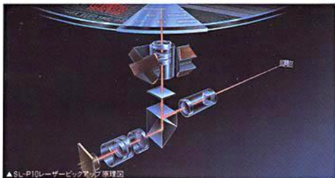
▲SL-P10レーザービックアップ 原理図
