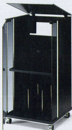
HS-X880 für „Midi“-Systeme 407 × 820 × 412 mm (B × H × T) max. Lichte Innenhöhe 484 mm
