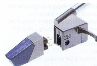
T4D-Steckanschlußsystem
