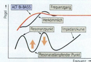
„Act Bi-Bass“-System
