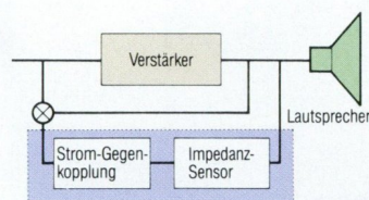
„Act Bi-Bass“-System
