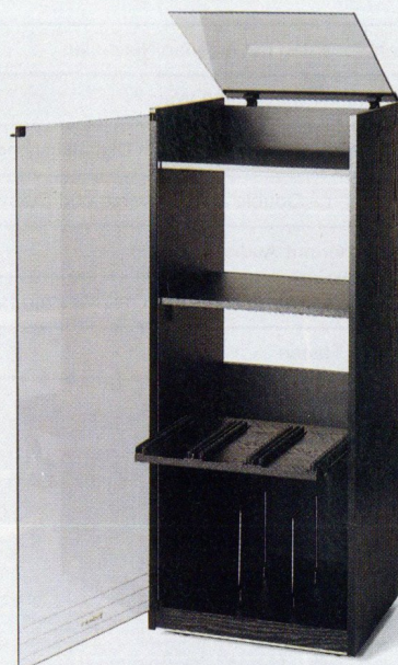
HS-605CD 476 × 1175 × 435 mm (B × H × T) max. Lichte Innenhöhe 768 mm
