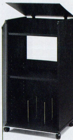
HS-625 473 × 920 × 440 mm (B × H × T) max. Lichte Innenhöhe 688 mm
