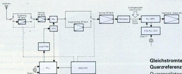
Blockdiagramm der ST-G90 Empfangsschaltung
