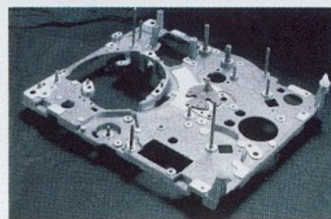
Aluminium-Druckgußchassis
