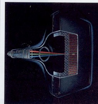
Die neue 70 cm Super-Quintrix Bildröhre
