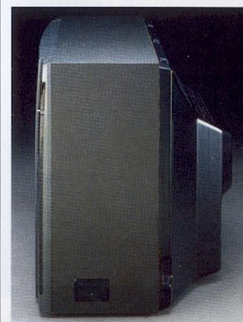
Die Seitenansicht des TX-2878 DRS mit der geringen Tiefe von 47 cm
