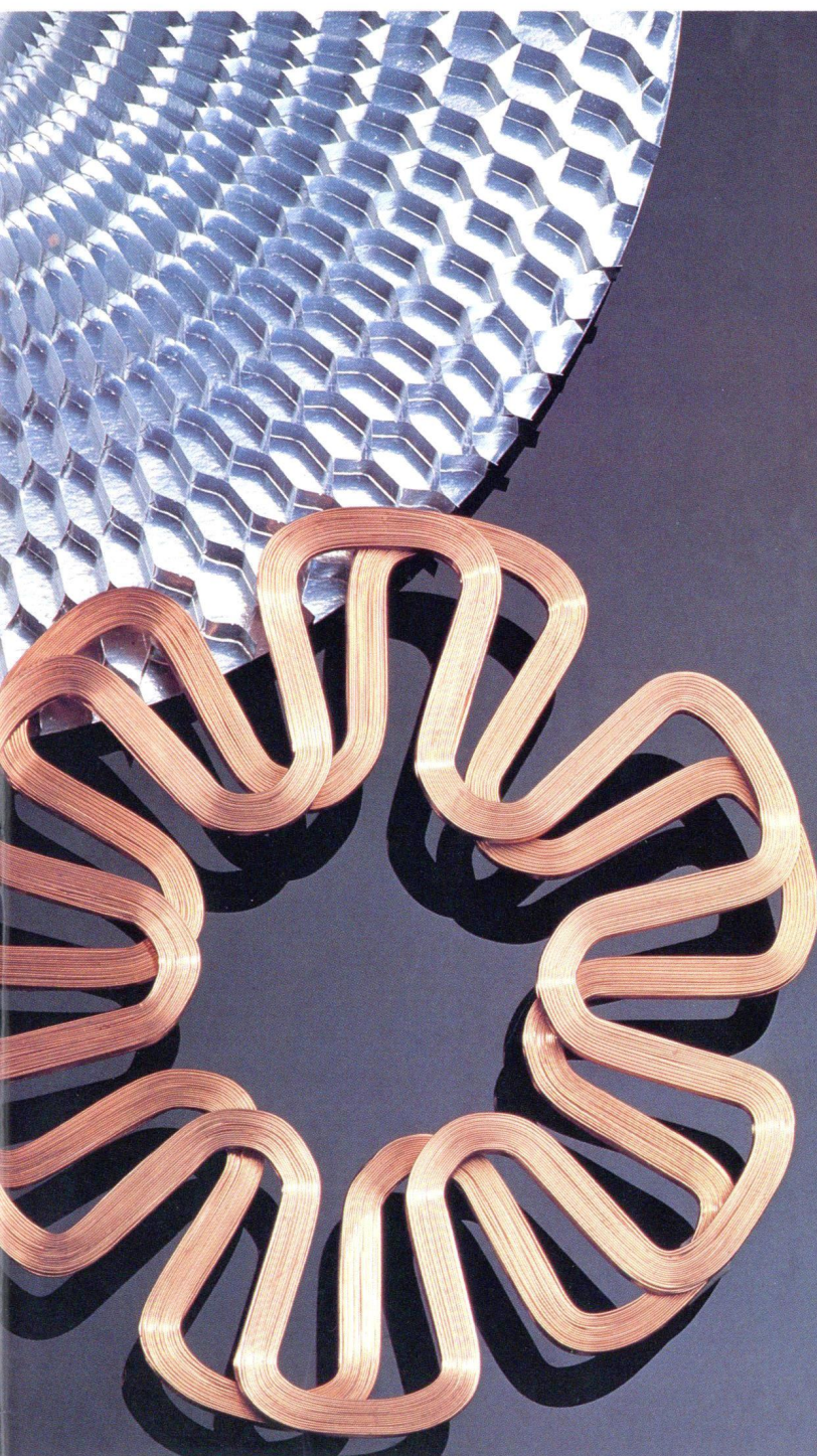
Spulenwicklung eines Direktantriebsmotors
