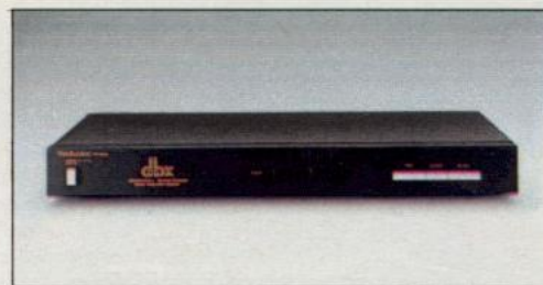
RP-9024 dbx-Rauschunterdrückungseinheit, Anschlußmöglichkeit an Cassettendecks, „dbx-disc“-Position – Möglichkeit der Decodierung von dbx-codierten Schallplatten. Dynamikumfang: 110 dB, Rauschabstand: 92 dB. Gehäusefarbe: schwarz.
