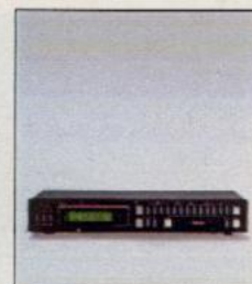
TE-96 Schaltuhr mit LCD-Anzeige. Schaltmöglichkeit: 4 Programme innerhalb 1 Woche über zwei unabhängige Stromkreise. Max. Anschlußlast: 1.100 W pro Stromkreis, Breite: 43 cm. Gehäusefarbe: schwarz.
