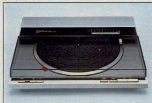
SL-QL1 Vollautomatischer Plattenspieler mit quarzgeregeltem Direktantrieb und Tangentialtonarm. Wiederholautomatik. Automatische Abtastung der Plattengröße. Hochwertiger Magnettonabnehmer EPC-P 22. Gleichlaufschwankungen \pm 0,035\% . Gehäusefarbe: schwarz + silber.
