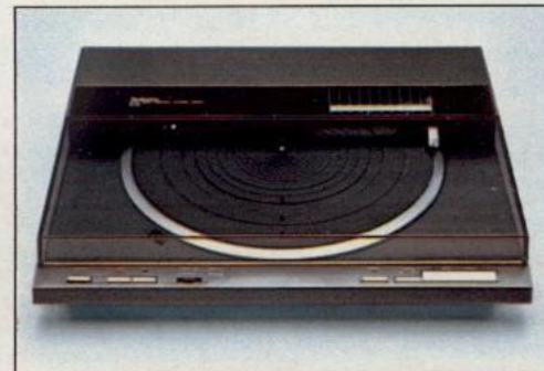
SL-DL1 Vollautomatischer Plattenspieler mit Direktantrieb und Tangentialtonarm. Wiederholautomatik. Automatische Abtastung der Plattengröße. Hochwertiger Magnettonabnehmer EPC-P 23. Geschwindigkeitsfeinregulierung \pm 5\% . Gleichlaufschwankungen \pm 0,055\% . Gehäusefarbe: schwarz + silber.
