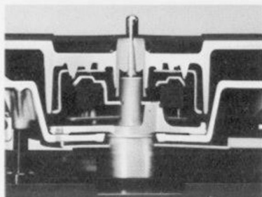
Schnittzeichnung von Modell SL-1300; deutlich sichtbar ist, daß der Plattenteller integraler Bestandteil (Rotor) des direktantriebenden Motors ist.
