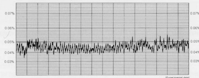
Gleichlaufschwankungen für RS-676USD, RS-671USD.
