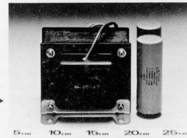
Leistungsstarker Netztransformator und extragroße Elektrolyt-Kondensatoren für Modell SA-5560.
