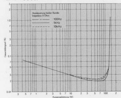
Ausgangsleistung und Klanggrad für SA-5560.
