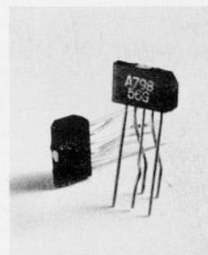
Abgestimmte Doppel-Transistoren in Einfananordnung in der Differentialverstärkerstufe jedes Kanals.
