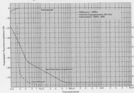
Eingangssignalpegel als Funktion des Ausgangspegels, Fremdspannungsabstand und Klanggrad (SA-5560).
