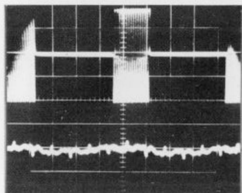
◀ Impulsverzerrungen in einem Kanal. Das Ausgangssignal wird nur an einen Kanal bei Tonbursts geliefert und die Impulsverzerrung in diesem Kanal gemessen.
