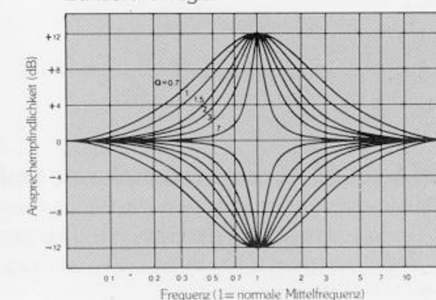
Bandbreitenregler
