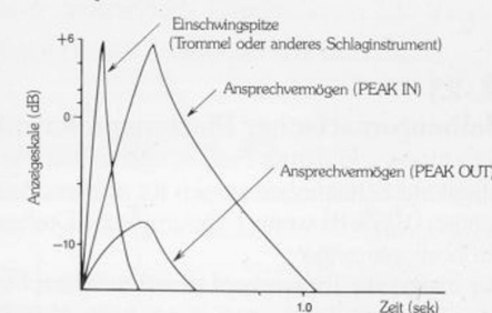
Spitzenwertkontrolle
