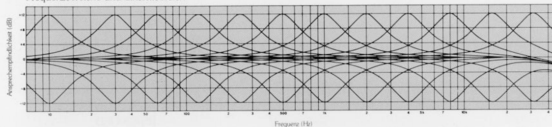
Regelumfang der Mittelfrequenz jedes Frequenzbereiches
