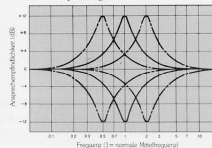
Mittelfrequenzregler
