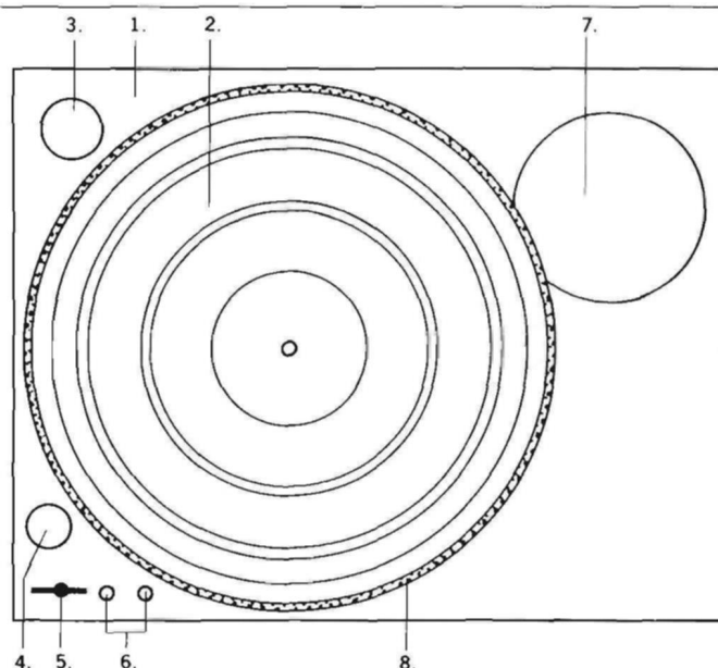
1. Chassis. 2. Pladetallerken. 3. Holder for 45-adaptér. 4. Stroboskoplampe. 5. Hastighedsomskifter. 6. Finjustering af hastighederne. 7. Monteringsplade for SME tonearm. 8. Stroboskopmarkeringer.
