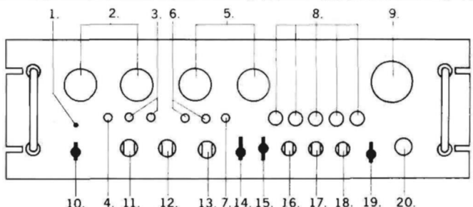
1. Kontrollampe. 2. Baskontroller for venstre og højre kanal. 3. Omskifter for baskontrollerens arbejdsfrekvens. 4. Udkobling af baskontrollerne. 5. Diskantkontroller for venstre og højre kanal. 6. Omskifter for diskantkontrollerens arbejdsfrekvens. 7. Udkobling af diskantkontrollerne. 8. Programvælger. 9. Styrkekontrol. 10. Afbryder. 11. Low filter. 12. High filter. 13. Funktionsomskifter. 14. Omskifter for båndkopiering. 15. Tape Monitor. 16. Impedansomskifter for Phono 1. 17. Impedansomskifter for Phono 2. 18. Følsomhedsomskifter for Phono 2. 19. Muting omskifter for 20 dB dæmpning af niveauet. 20. Balancekontrol.
