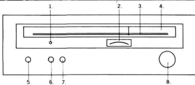
1. Kontrollampe for FM-stereo. 2. Midtpunktsinstrument for FM/feltstyrkeinstrument for AM. 3. Stationsskala AM. 4. Stationsskala FM. 5. Afbryder. 6. Programvælger. 7. Muting. 8. Skalaknap.
