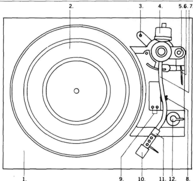
1. Chassis. 2. Pladetallerken. 3. Holder for 45-adapter. 4. Kontravægt. 5. Antiskating. 6. Pick-up lift. 7. Tonearm. 8. Tonearmholder. 9. Justeringsskruer for hastighederne. 10. Pick-up hus. 11. Omløber. 12. Hastighedsomskifter.
