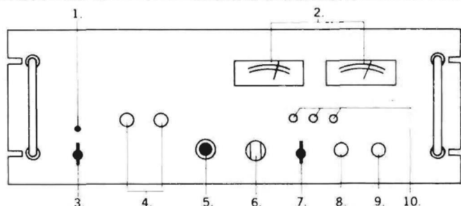
1. Kontrollampe. 2. Spidsværdiende instrumenter for udgangseffekt. 3. Afbryder. 4. Højttaleromskifter. 5. Hovedtelefonbøsning. 6. Omskifter for udgangsimpedans. 7. Afbryder for det tilførte signal. 8. Niveauekontrol for venstre kanal. 9. Niveauekontrol for højre kanal. 10. Følsomhedsomskiftere for instrumenterne.
