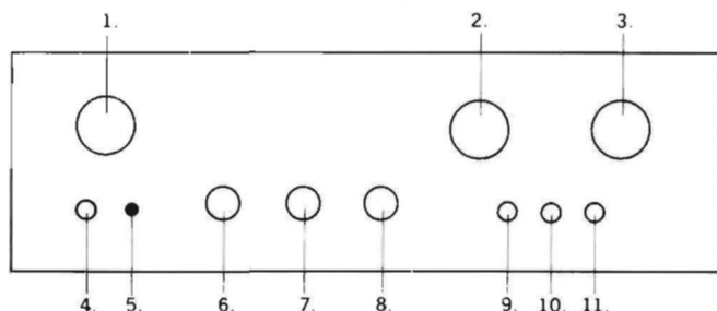
1. Højttaleromskifter. 2. Styrkekontrol. 3. Programvælger. 4. Afbryder. 5. Hovedtelefonbøsning. 6. Baskontrol. 7. Diskantkontrol. 8. Balancekontrol. 9. Loudness. 10. Mono/stereoomskifter. 11. Tape Monitor knap.
