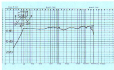
Der Frequenzgang der SC 40
