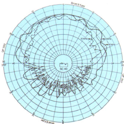
Die Abstrahl-Charakteristik der SC 40
