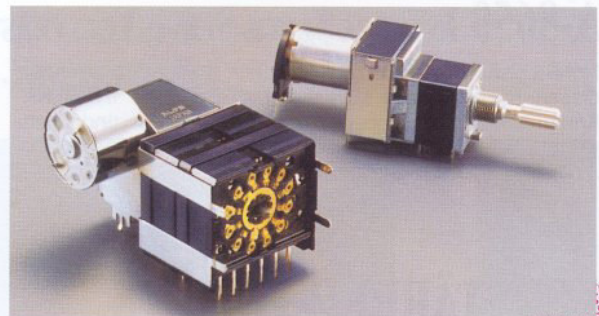
Logic-Controlled Motor-Selector und motorgesteuerter Lautstärkereglern.
