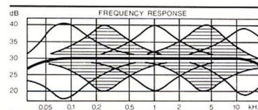
Frequenzgang und Wirkungsweise des Equalizers.
