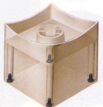
Konstruktion des Standfußes mit resonanzabsorbierenden Füßen.
