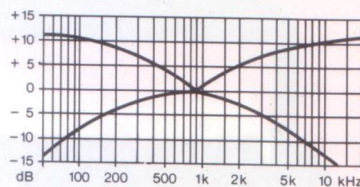
Frequenzgang und Wirkungsweise der beiden Klangregler.
