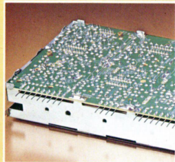
Abbildung links: PAL/Secam-Decoder (CCIR) zum Empfang von DDR-Farbfernseh-Programmen (Austauschmodul).
