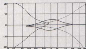
Wirkungsweise des 3-fach Klangregel-Netzwerkes.
