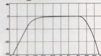
Wirkungsweise von Rausch- und Rumpelfilter.
