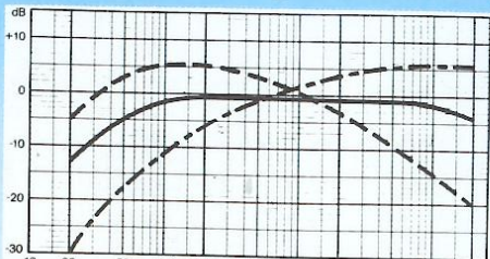
Frequenzgang bei — Mittelstellung - - - Bassregler auf · Höhenregler zu ····· Bassregler zu · Höhenregler auf gemessen nach DIN 45 500.
