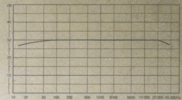
Leistungsbandsbreite
