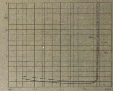
Klirrfaktor
