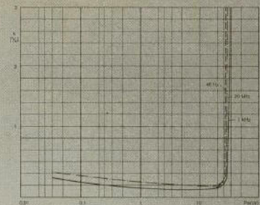
Klirrfaktor
