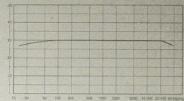
Leistungsbandbreite
