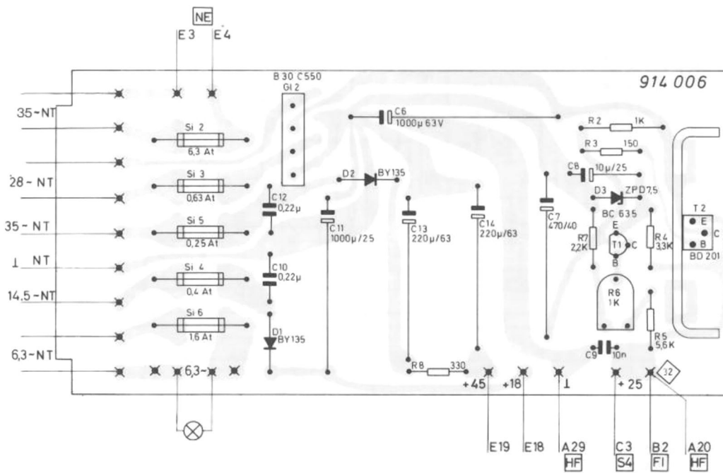
N-Platine auf die Bestückungsseite gesehen
