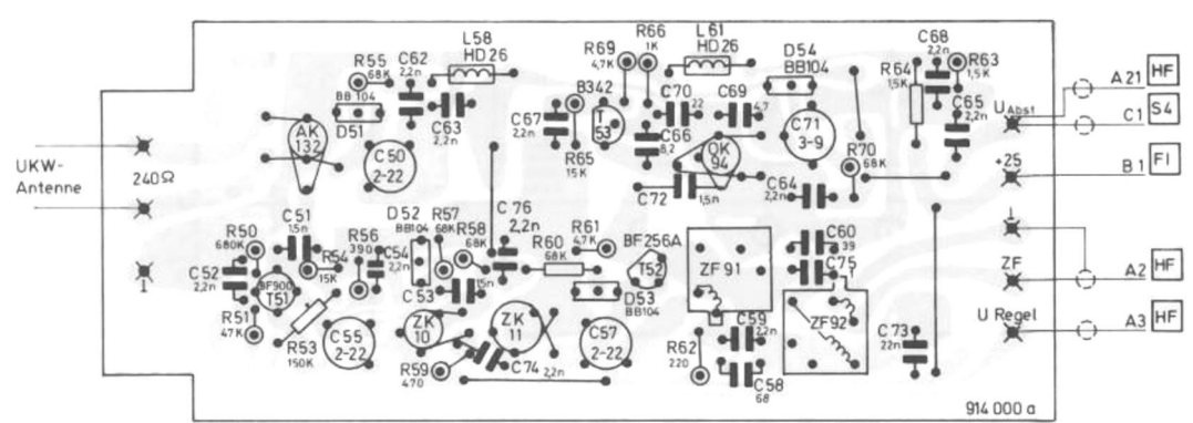
U-Platine auf die Leiterseite gesehen
