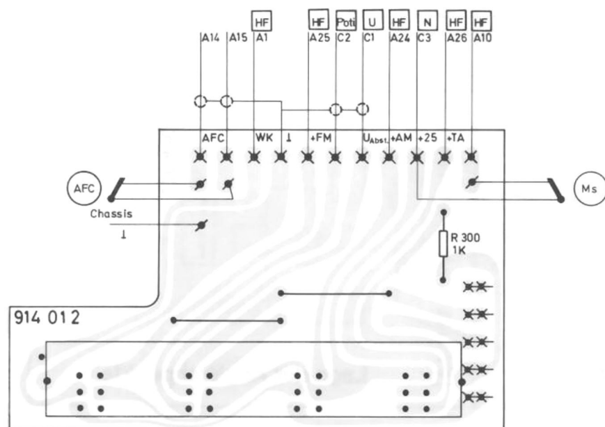
Ansicht Speicher-Baustein
