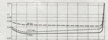
Klirrfaktor in Abhängigkeit von der Aussteuerung bei 40 Hz, 1 kHz und 12,5 kHz.
