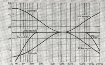
Frequenzgang in Stellung Linear und mit eingeschaltetem Rausch- und Rumpelfilter. Regelbereich der Baß- und Höhenregler.
