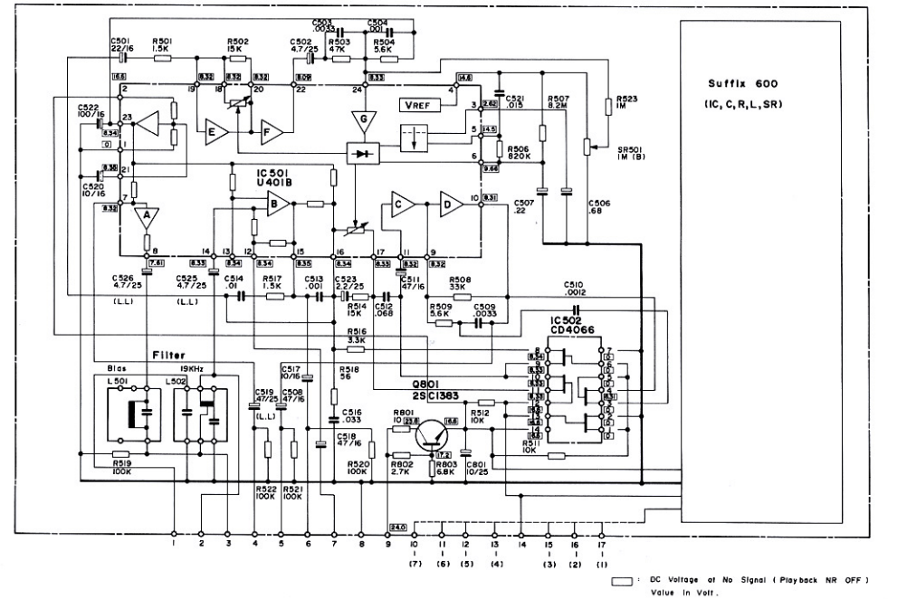
SCHALTBILD HIGH-COM (AUFNAHME)
