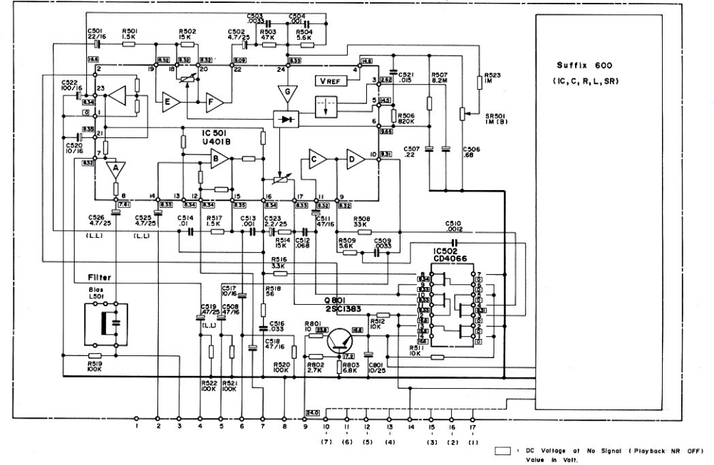
SCHALTBILD HIGH-COM (AUFNAHME)
