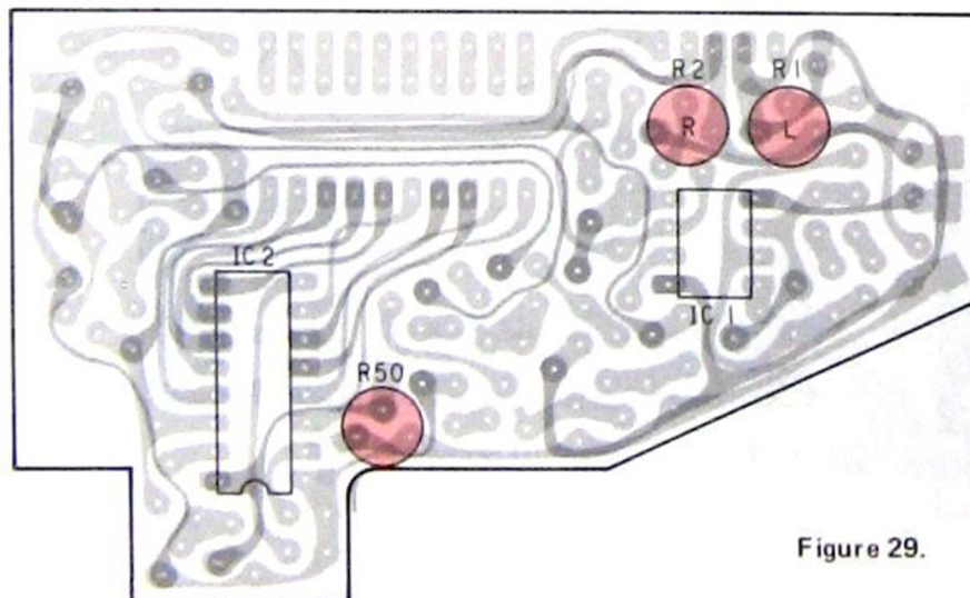
Meter Drive P.C.Board
