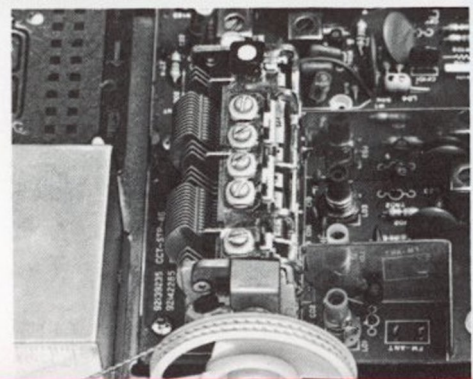
Der 4-fach-Drehkondensator trägt zu den überragenden Empfangsqualitäten des SA 620 und SA 520 entscheidend bei.
