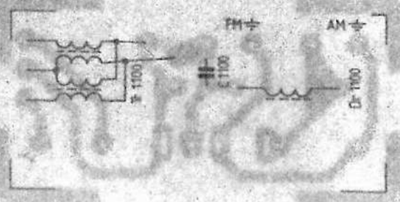
Antennenplatte 7 815 050
