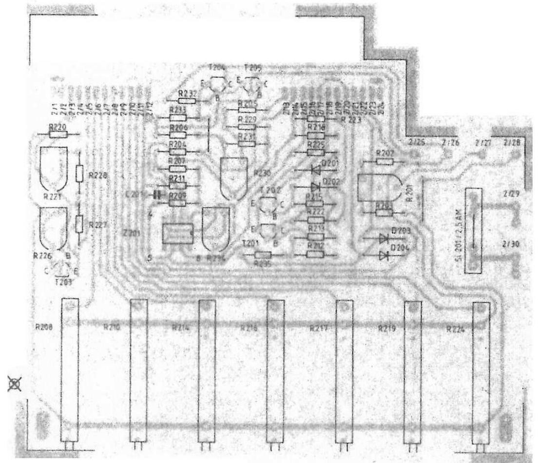
Festsenderplatte 7 815 006
