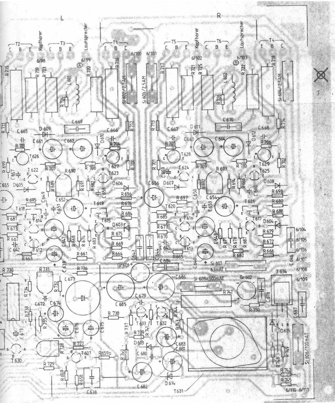
Endstufenplatte 7 815 010
