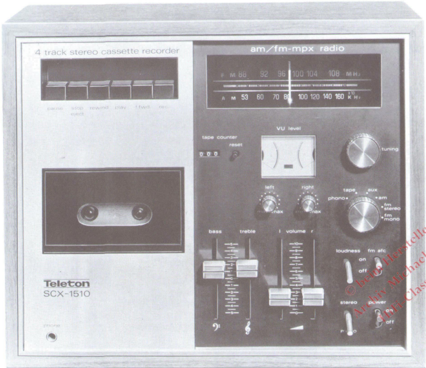
SCX 1510 Kompaktanlage mit Tuner, Verstärker und Cassettenrecorder UKW + MW Empfangsbereiche Verstärker mit 2x10 W Sinus Stereo Cassetten Recorder für Aufnahme und Wiedergabe Anschlüsse für Plattenspieler mit magn. Tonabnehmer, Mikrofone, sonst. Tonquellen, 2 Boxen und Kopfhörer Abmessungen 350x310x170 mm
