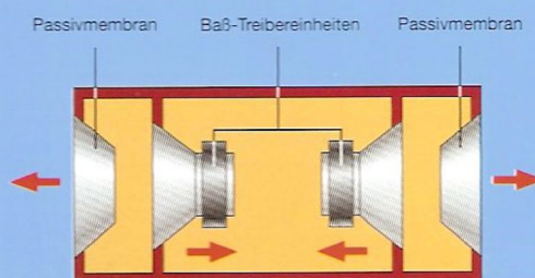
D.D.D.-Lautsprecher System
