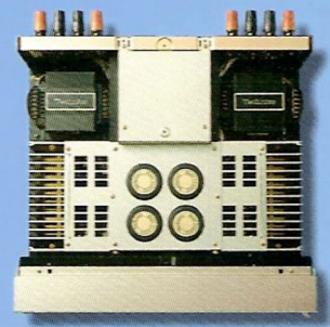
Sauberer Twin-Monorial Aufbau der Endstufe
