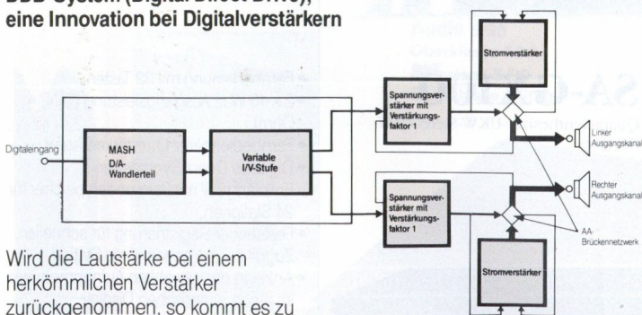
DDD-System, Blockdiagramm
