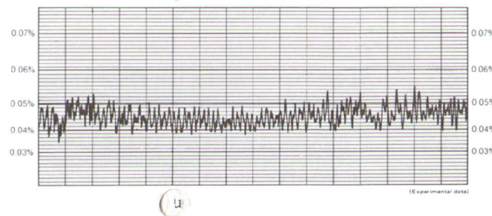
Gleichlaufschwankungen für RS-676USD, RS-671USD.
