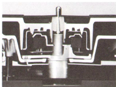
Schnittzeichnung von Modell SL-1300; deutlich sichtbar ist, daß der Plattenteller integraler Bestandteil (Rotor) des direktantreibenden Motors ist.
