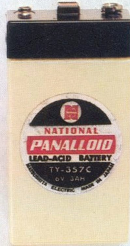
TY-357 C Akku für TR-499 EU und TR-475 EU.
