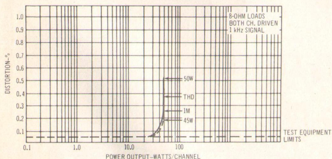
Fig. 5—THD and IM characteristics.
