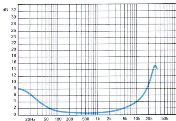
Aufnahme-Kurve 19 cm/s
