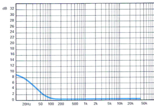
Aufnahme-Kurve 38 cm/s
