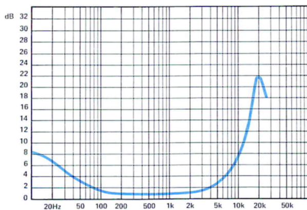
Aufnahme-Kurve 9,5 cm/s
