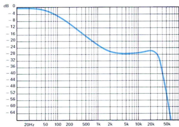
Wiedergabe-Kurve 9,5 cm/s
