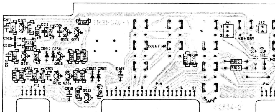
A3 OUTPUT MIC/LINE AMP.
