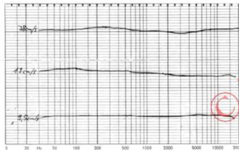
fig. 1. Frekwentieverloop bij weergave voor de 3 bandsnelheden.
