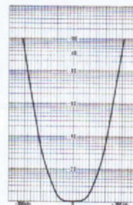
Følsomhetskurver for FM-mottakeren i mono og stereo.
