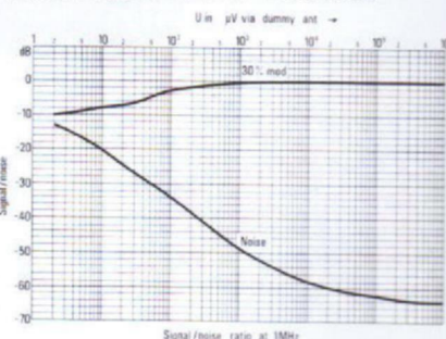
Følsomhetskurve for AM-mottakeren.
