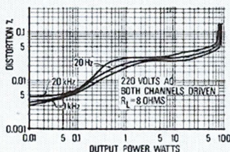
Vervorming als functie van het uitgangsvermogen (beide kanalen regelijk).
