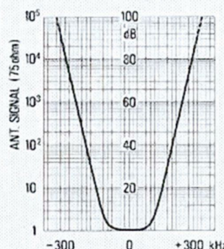
Selectiviteits karakteristiek van de FM-ontvanger.
