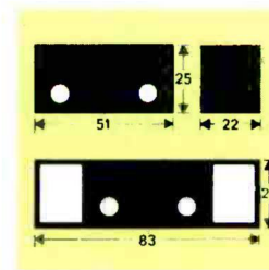
Croquis de dimensiones. En la parte superior: Huldra 8-55, en la inferior: Huldra 8-56. Mueble en caja de teca con elegante acabado.
