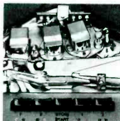
3 cabezas sonoras para supresión, grabación y reproducción, de fabricación Tandberg.
