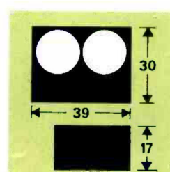
Croquis de dimensiones Caja en madera de teca con elegante acabado.
