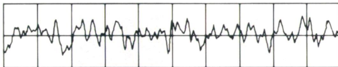
Servo-Steuersignal mit S-Servo III.
