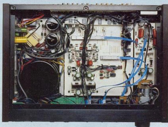
High-End-Vorverstärker TA-E 77 ESD mit Digitaleingängen und Digitalausgang zur Kommunikation mit anderen digitalen Medien.
