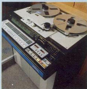
Die Sony 24-Kanal-Maschine PCM-3324 für Mehrkanalaufzeichnung einzelner Instrumente und Stimmen.
